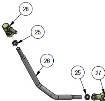
035-5451-00 Push Rod-Left
