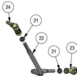
035-5450-00 Push Rod-Right
