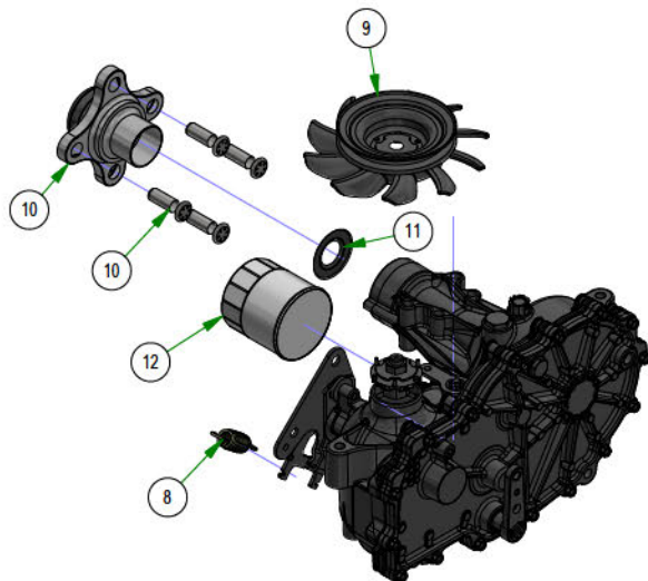
050-2095-03 2025 RH 3100 Transaxle
