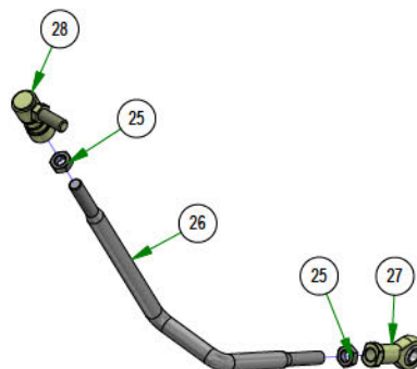
035-5451-00 Push Rod-Left
