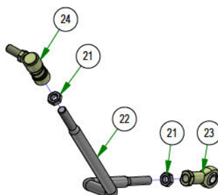
035-5450-00 Push Rod-Right
