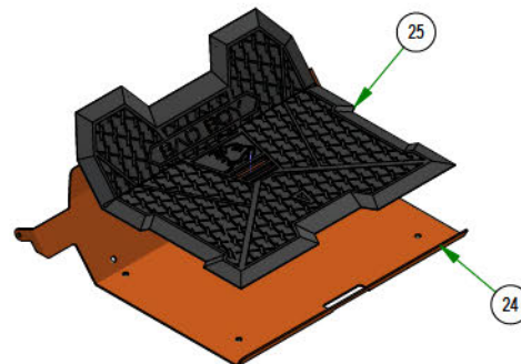
079-3155-24 FLOORBOARD ASSEMBLY
