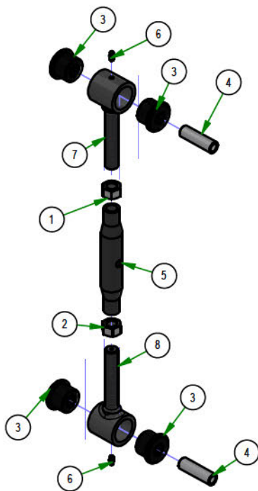
048-9000-00 Turnbuckle
