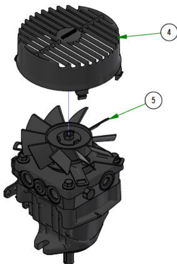
050-3001-00 & 050-3003-00 PUMP ASSEMBLIES
