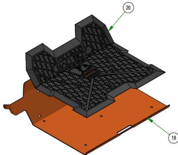
079-3155-24 FLOORBOARD ASSEMBLY
