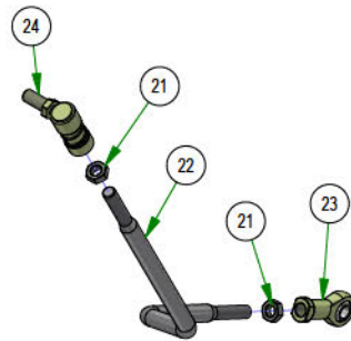
035-5450-00 Push Rod-Right
