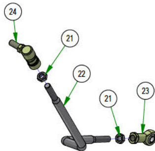
035-5450-00 Push Rod-Right
