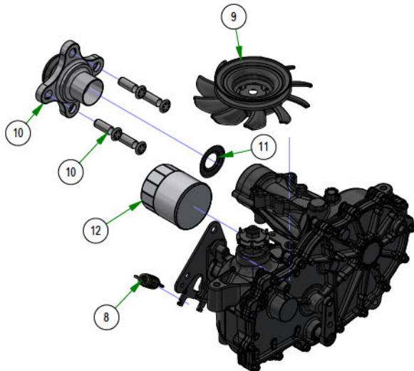
050-2095-03 2025 RH 3100 Transaxle
