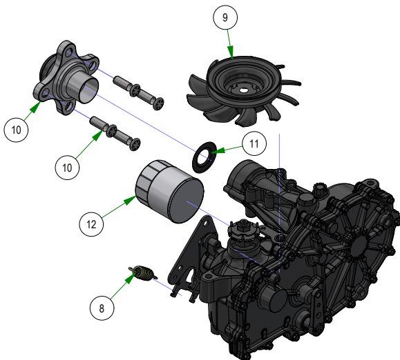
050-2095-03 2025 RH 3100 Transaxle
