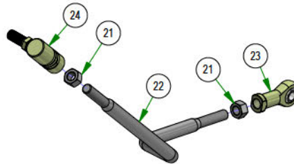
035-5450-00 Push Rod-Right
