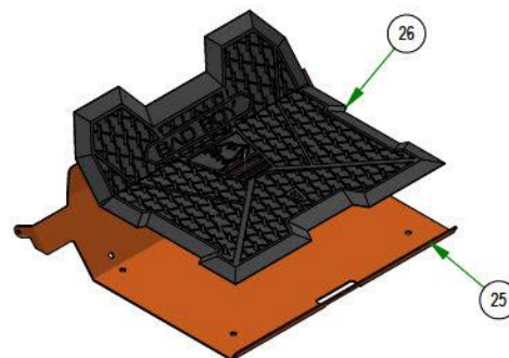
079-3155-24 FLOORBOARD ASSEMBLY
