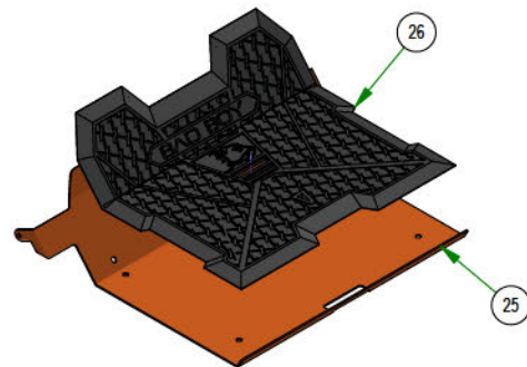
079-3155-24 FLOORBOARD ASSEMBLY
