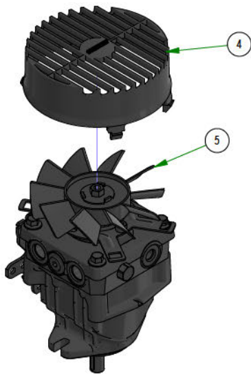
050-3001-00 & 050-3003-00 PUMP ASSEMBLIES
