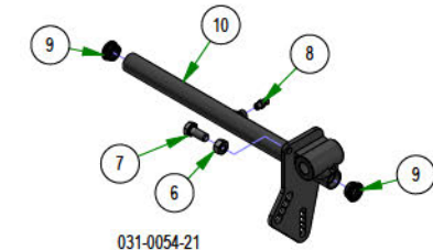
031-0054-21 2021 Maverick Drive Arm Actuator LH Assembly
