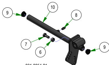
031-0054-21 2021 Maverick Drive Arm Actuator LH Assembly
