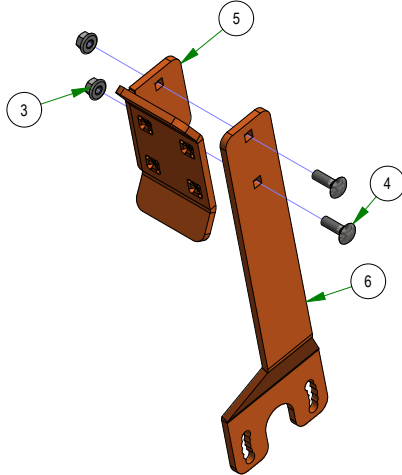
026-0019-01 Foot Pedal Assembly
