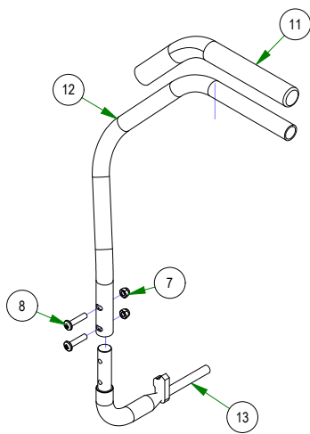
031-8851-70 ZT Steering Arm, Right Hand
