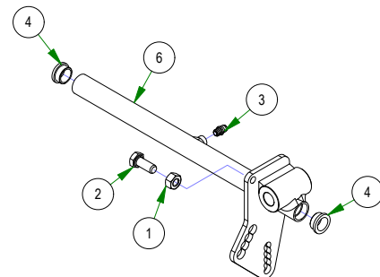
031-0054-21 2021 Maverick Drive Arm Actuator LH Assembly
