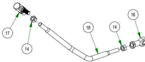
035-5451-00 Push Rod - Left
