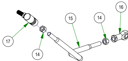
035-5450-00 Push Rod - Right
