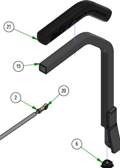
031-9071-00 LEFT DRIVE ARM
