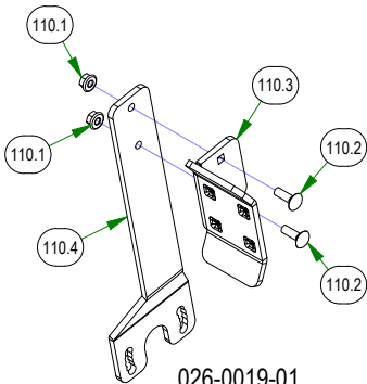
026-0019-01 Foot Pedal Assembly
